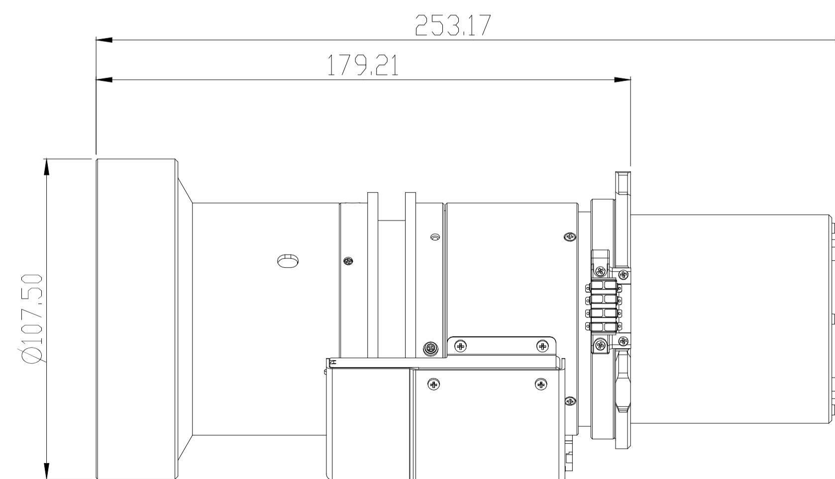
TR 2.00~4.00 LONG ZOOM (BX-CTA22)
