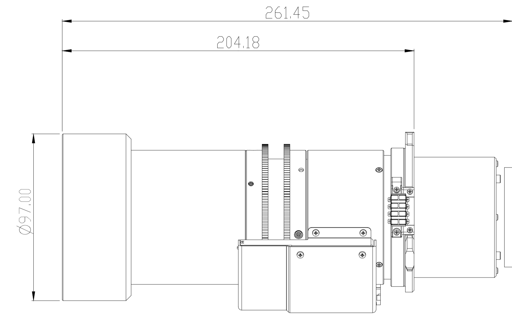
TR 4.00~7.20 ULTRA LONG ZOOM (BX-CTA23)
