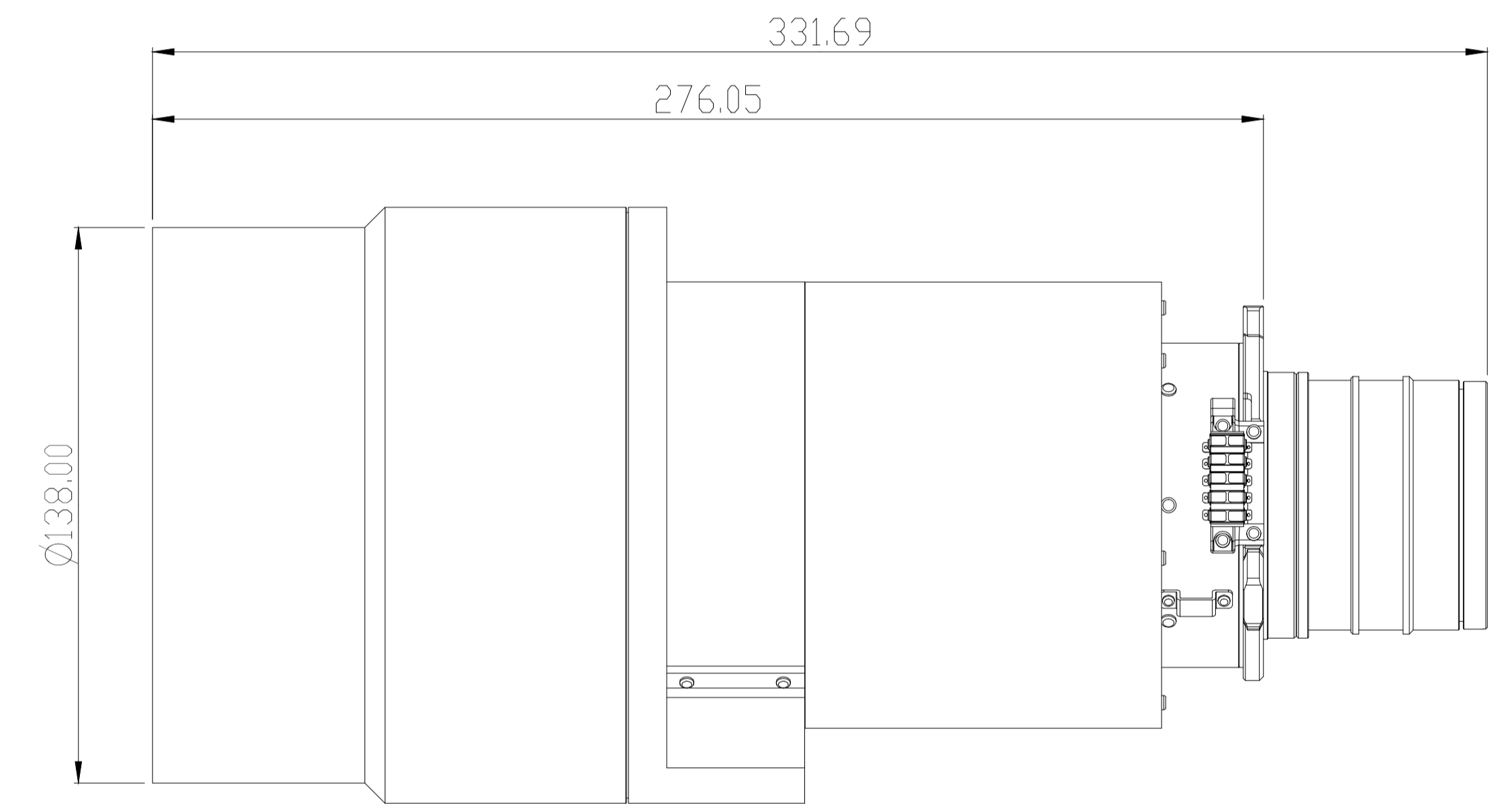
TR 7.20~10.8 ULTRA LONG ZOOM (BX-CTA27)
