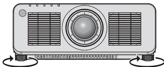
Maximal einstellbarer Bereich Einstellbare FüÙe: je 30 mm (1-3/16")
