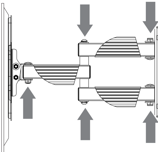
Gelenkbeweglichkeit anpassen Adjust hinge mobility
