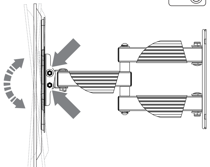
Neigung anpassen Adjust inclination
