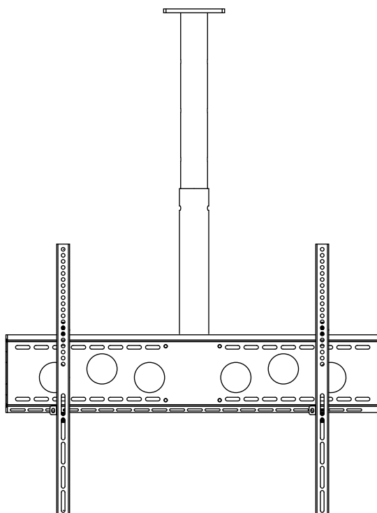
HA DH 400 - 700 L Art.-Nr. / Item no.: 2703
