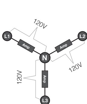
3 phase Y 120V
