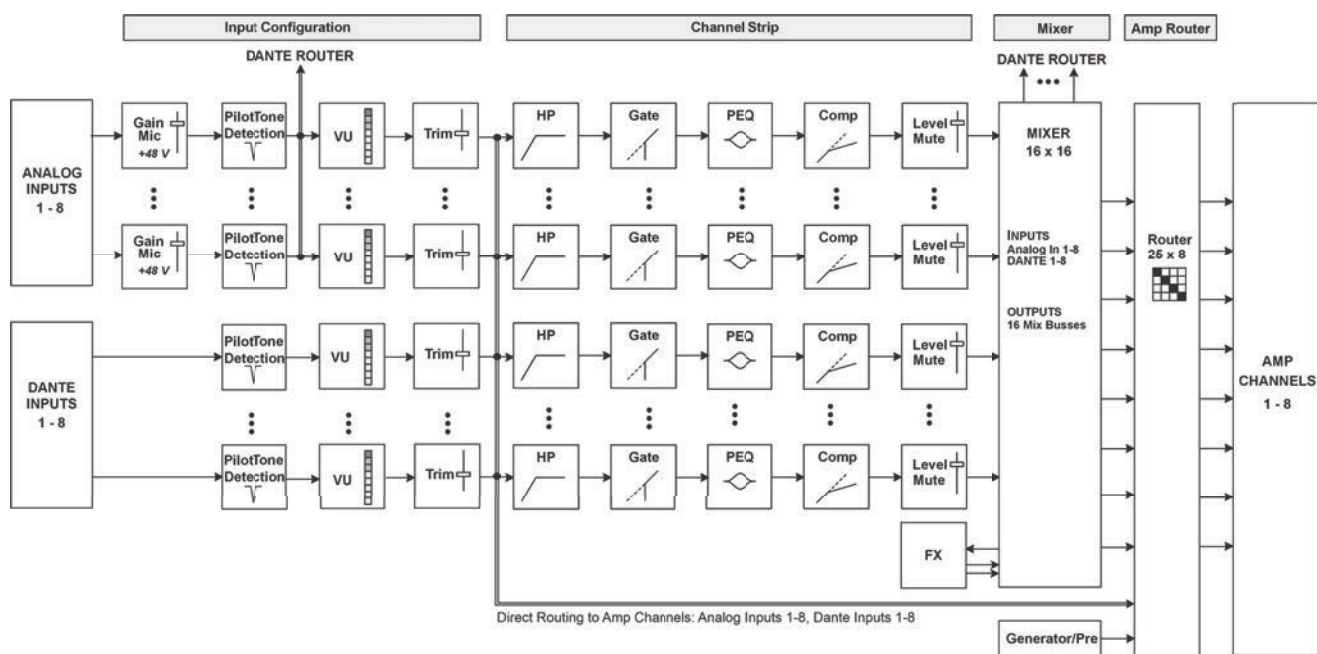
Abbildung 6.1: Eingangsblockdiagramm
