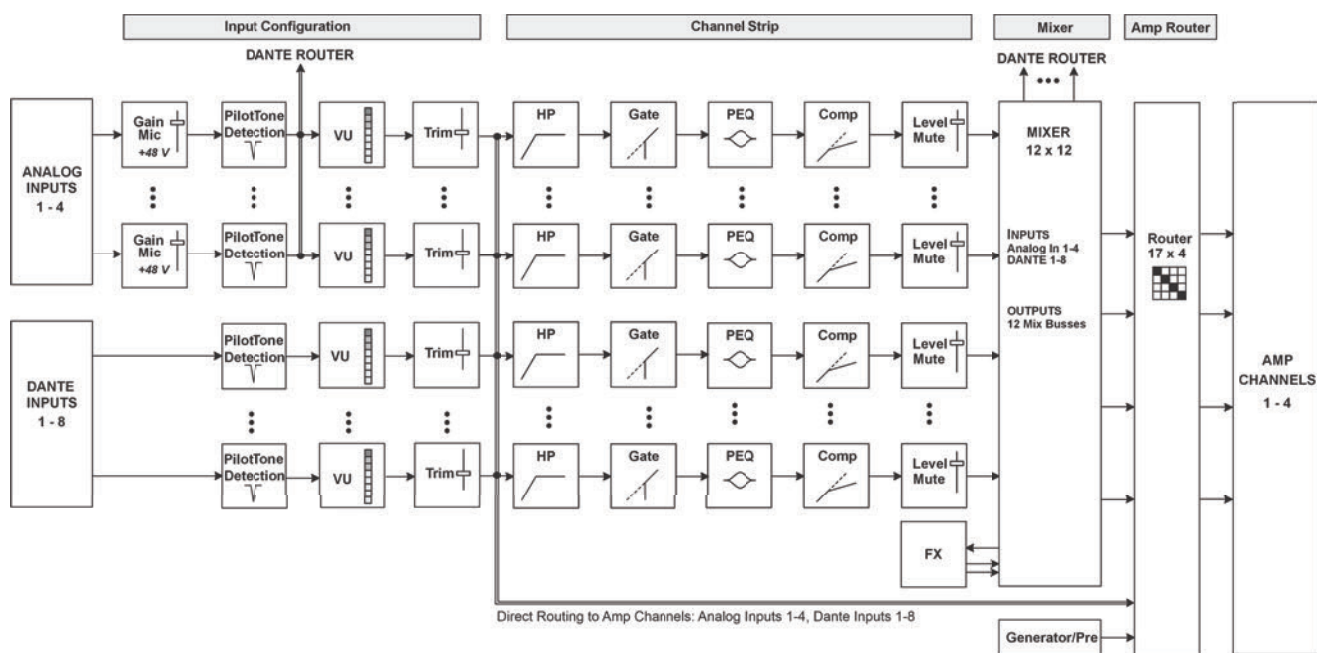
Abbildung 6.2: Eingangsblockdiagramm
