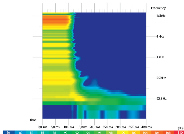
Spektrogramm
